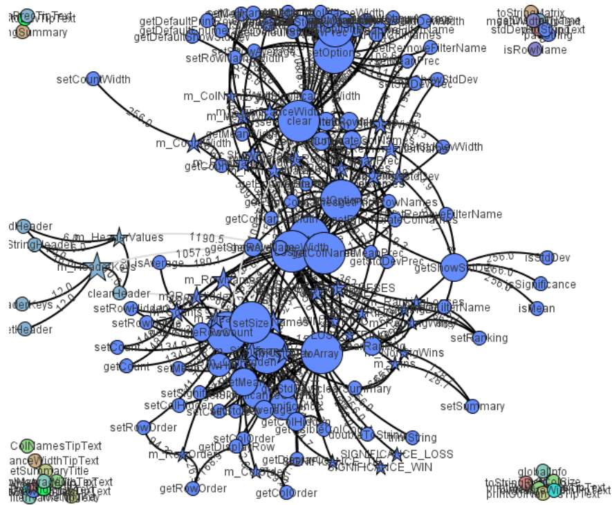
(a) Ungrouped
