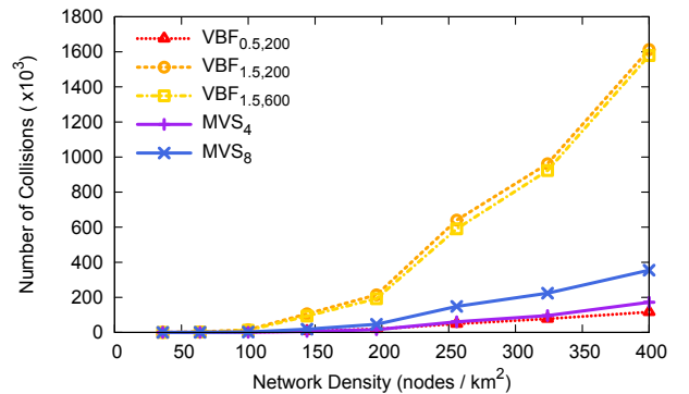
(d) Number of Collisions vs Network Density
